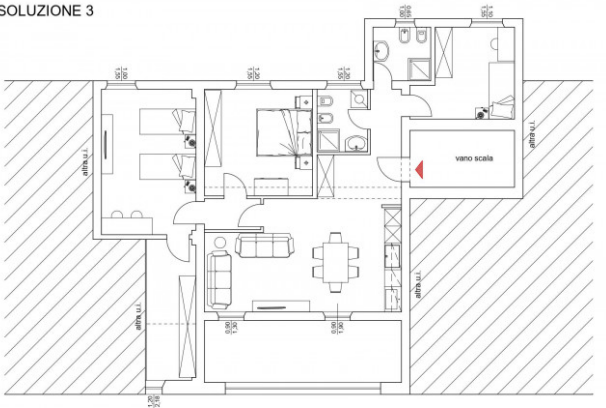
Pianta piano quarto
