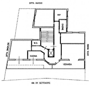
- PIANTA PIANO QUINTO - H=3.00m -
